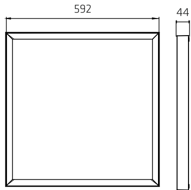
LUMINAIRE DIMENSIONS
